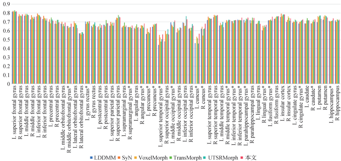
图7 不同方法在LPBA40每个解剖结构的Dice值
