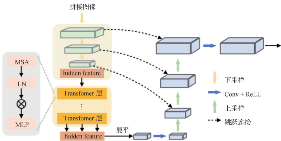
图3 保真项模块网络架构 Fig. 3 Network architecture of the fidelity module
