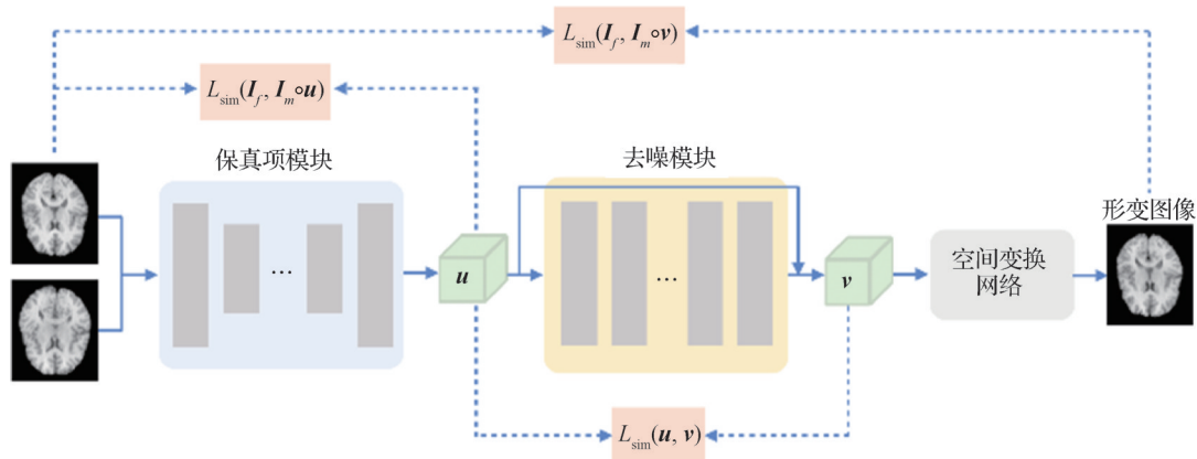
图2 深度展开配准网络单阶段流程
