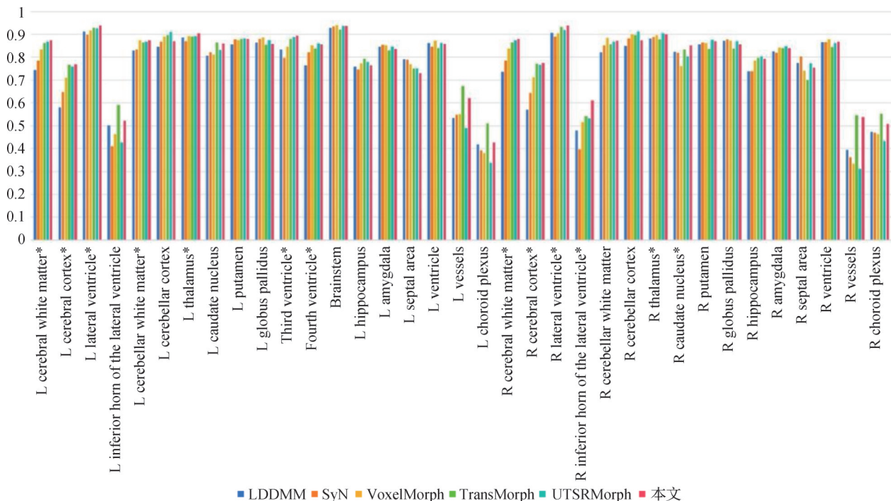
图8 不同方法在OASIS每个解剖结构的Dice值
