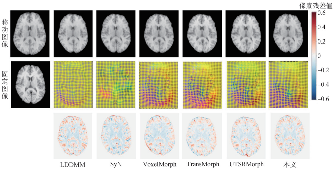
图5 不同方法在LPBA40数据集的可视化结果
